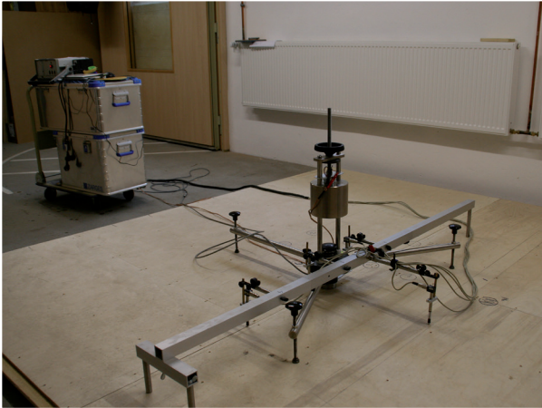
Messung der Standardverformung eines Sportbodens
