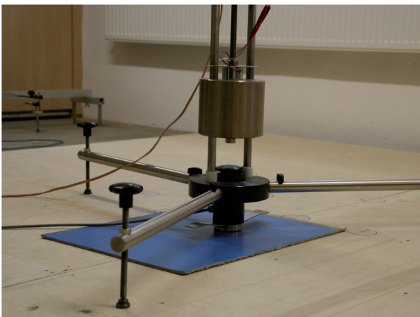
Messung des Kraftabbaus eines Sportbodens
